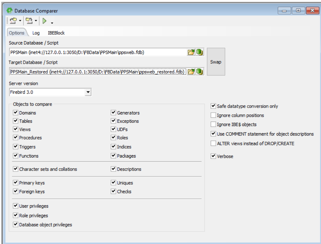
Рисунок 6.12 Параметры сравнения структуры
