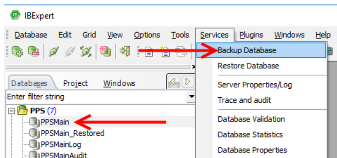
Рисунок 6.5 Архивирование базы данных
