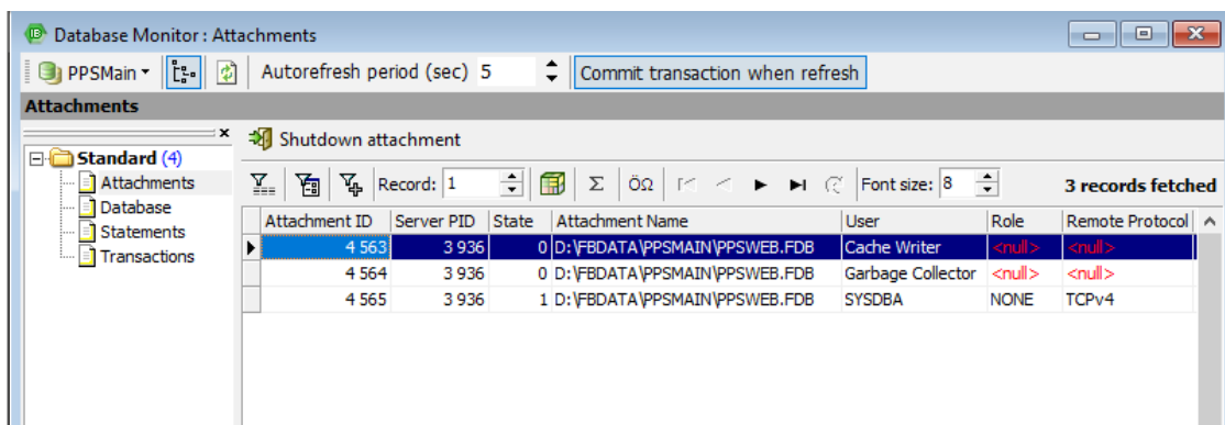
Рисунок 6.4 Мониторинг активности пользователей
