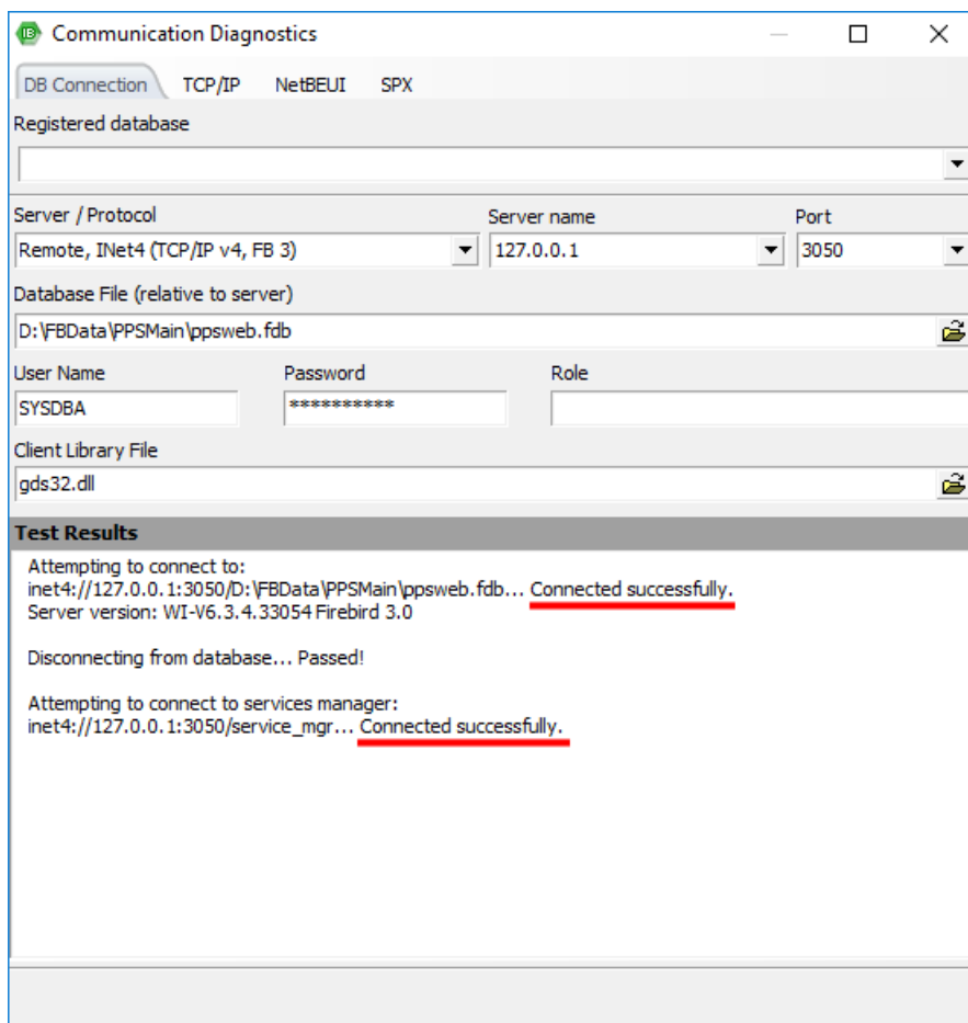
Рисунок 6.3 Проверка подключения к базе данных
