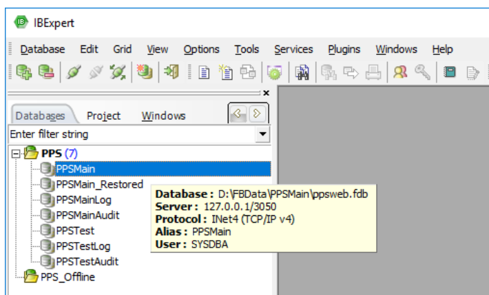
Рисунок 6.1 Список соединений в IBExpert
